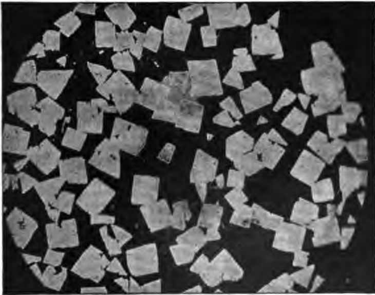
Fig. 37. Alloy of 80 per cent Tin, 20 per cent Antimony.
